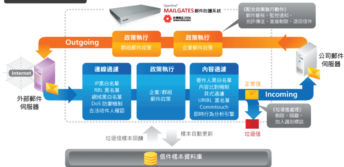
MailGates 過濾流程圖
